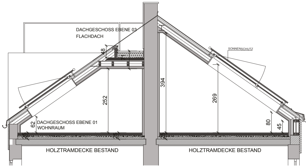
SCHNITT HOFTRAKT DACHFLÄCHENFENSTER
