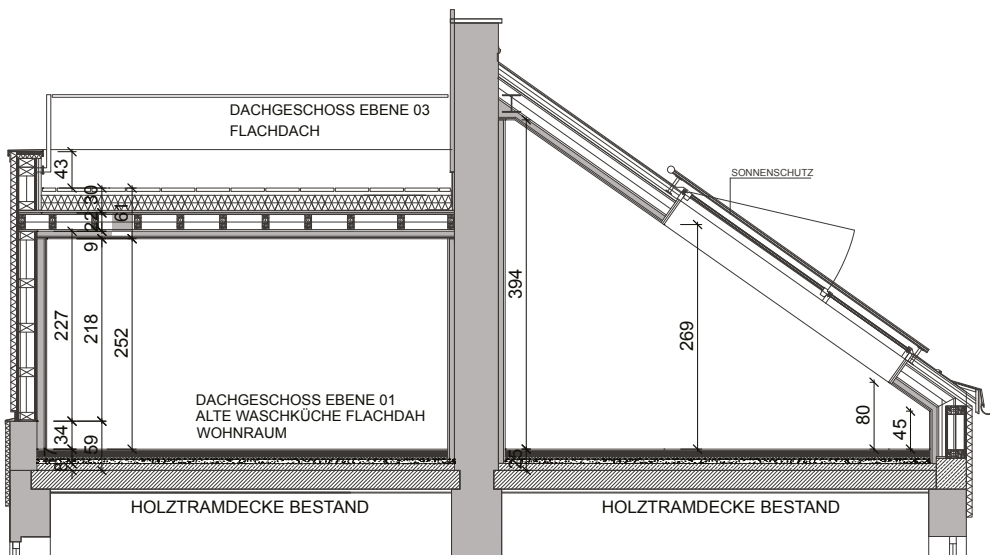
SCHNITT HOFTRAKT FLACHDACH
